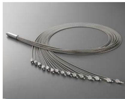
多分岐バンドルファイバ
